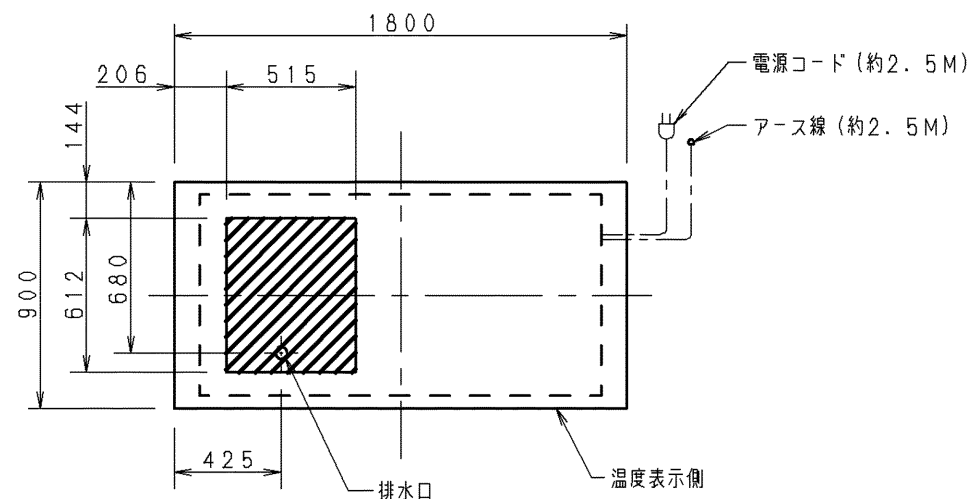
上面投影図 (SCALE 1/30)
