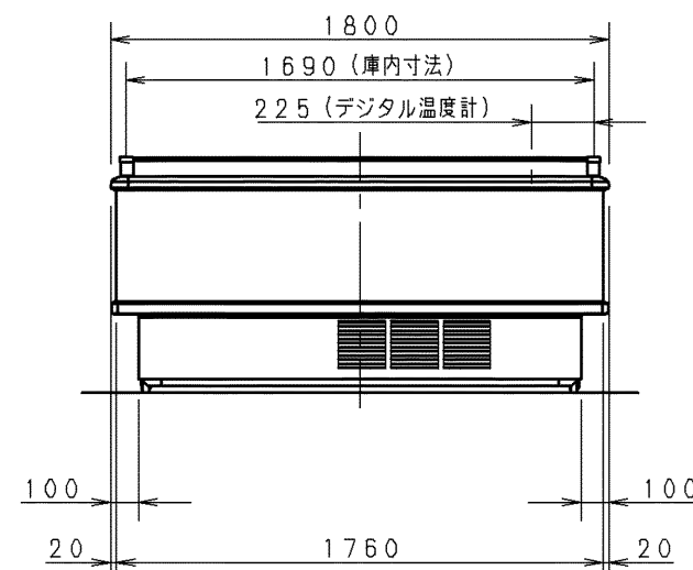
正面図 (SCALE 1/30)
