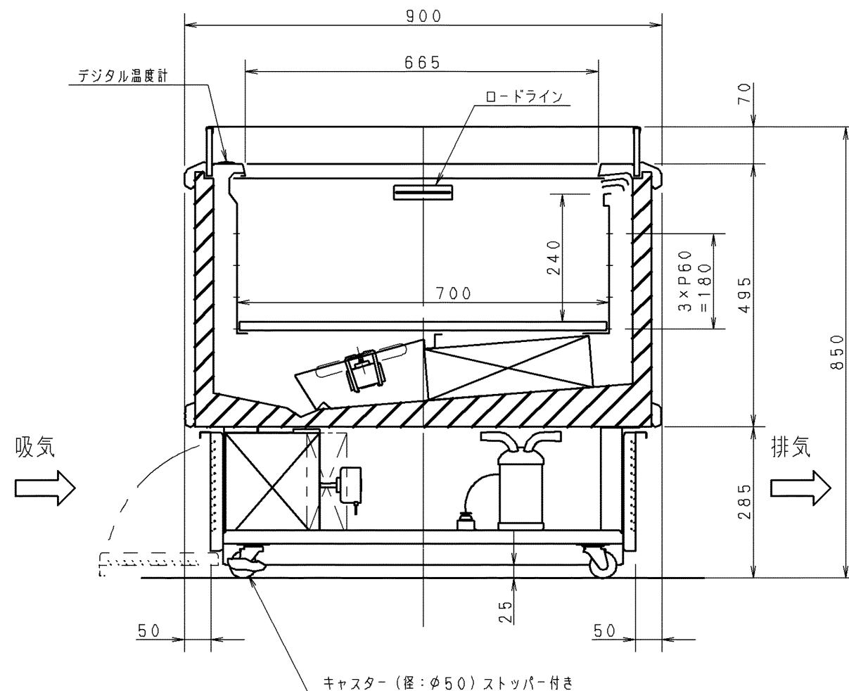
正面図 (SCALE 1/30)
