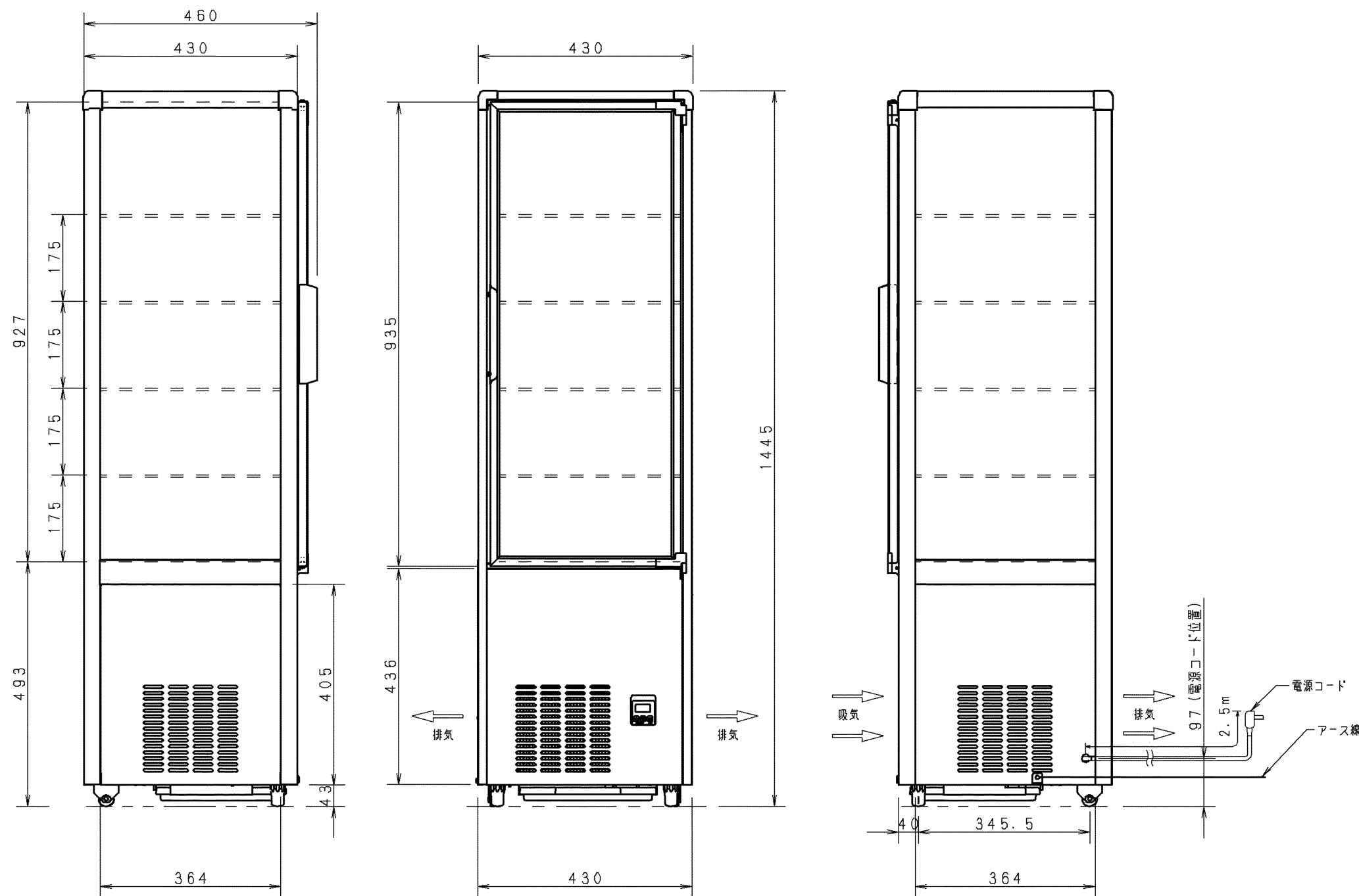
陳列部寸法
