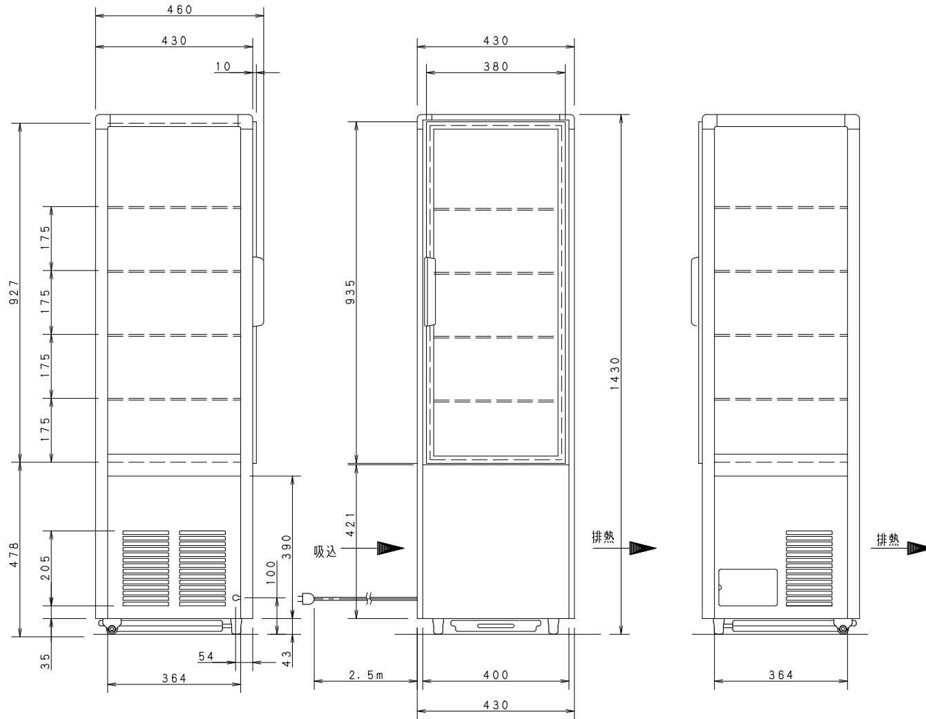
陳列部寸法
