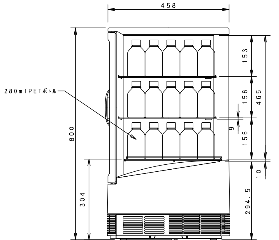
SMR-C65F取付例(取付時有効内容積59L)
