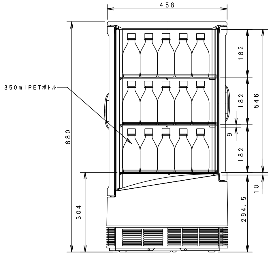
SMR-C75取付例(取付時有効内容積69L)
