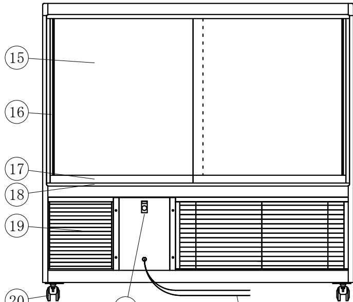
(A矢視図)
