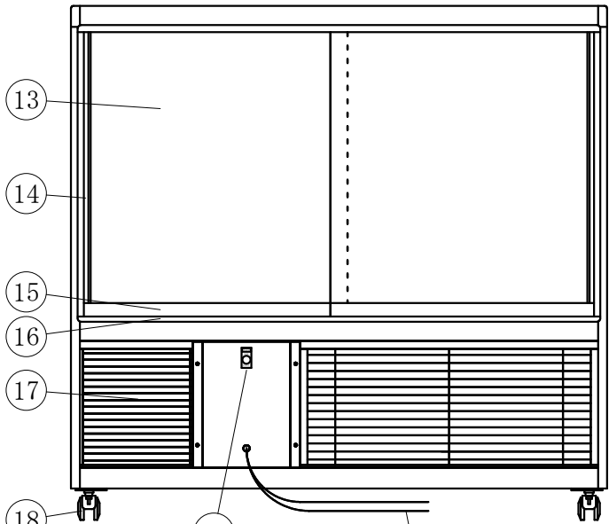
(A矢視図)
