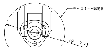
キャスター回転範囲 (SCL=1/2)
