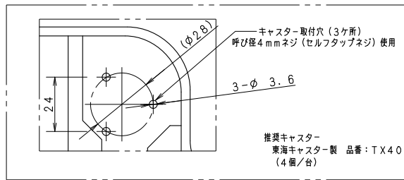
キャスター取付用 参考寸法図 (SCL=3/5)
