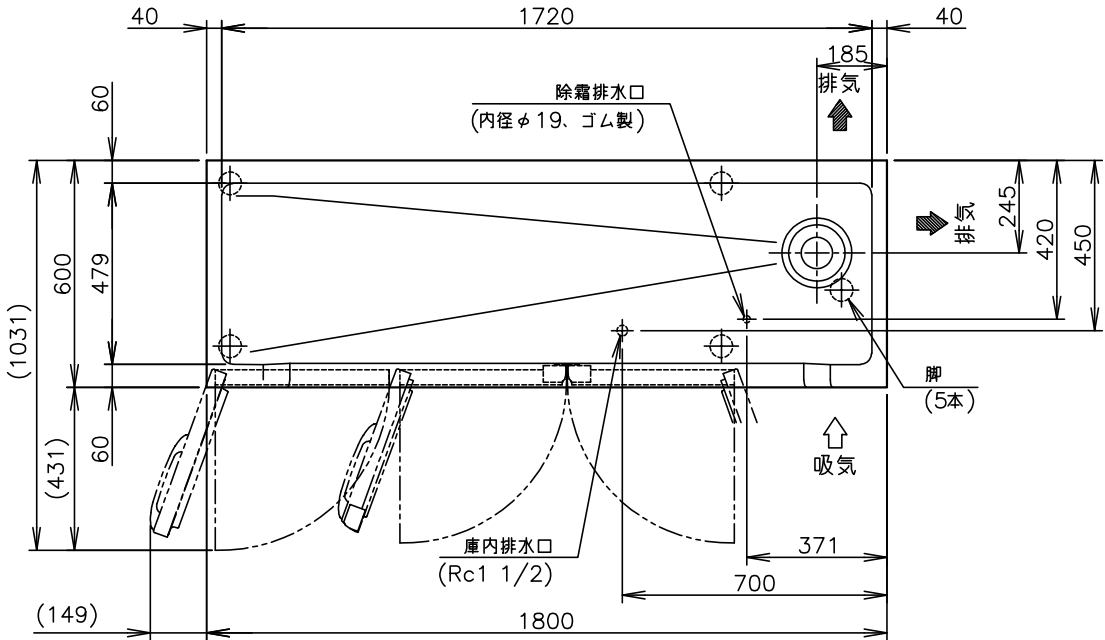
B矢视图(1/10)
