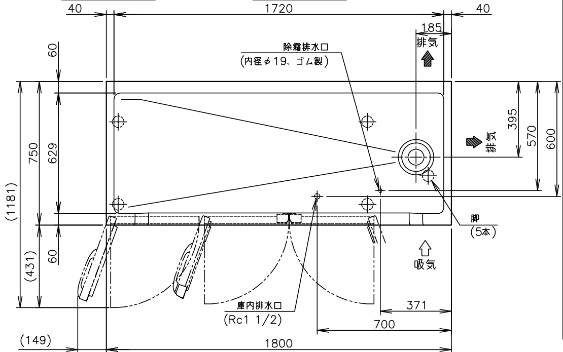
B矢視図(1/10)
