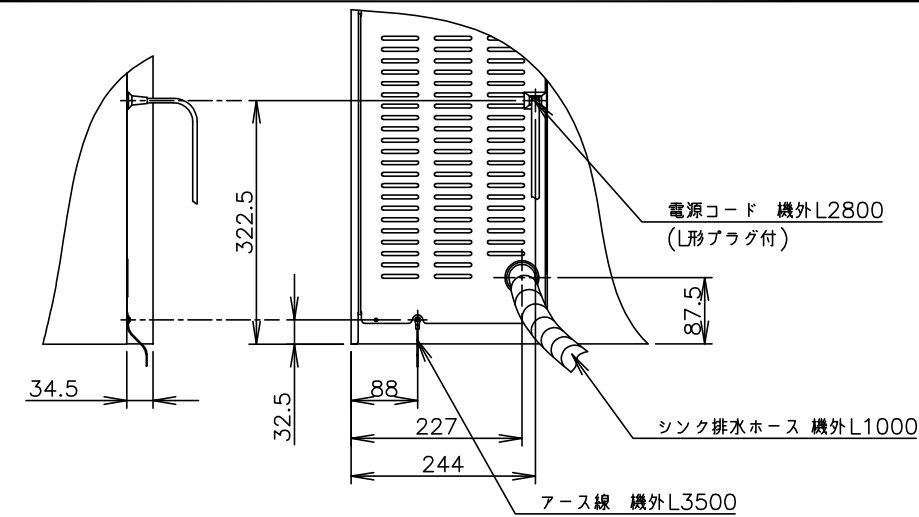
B矢視図(1/10)
