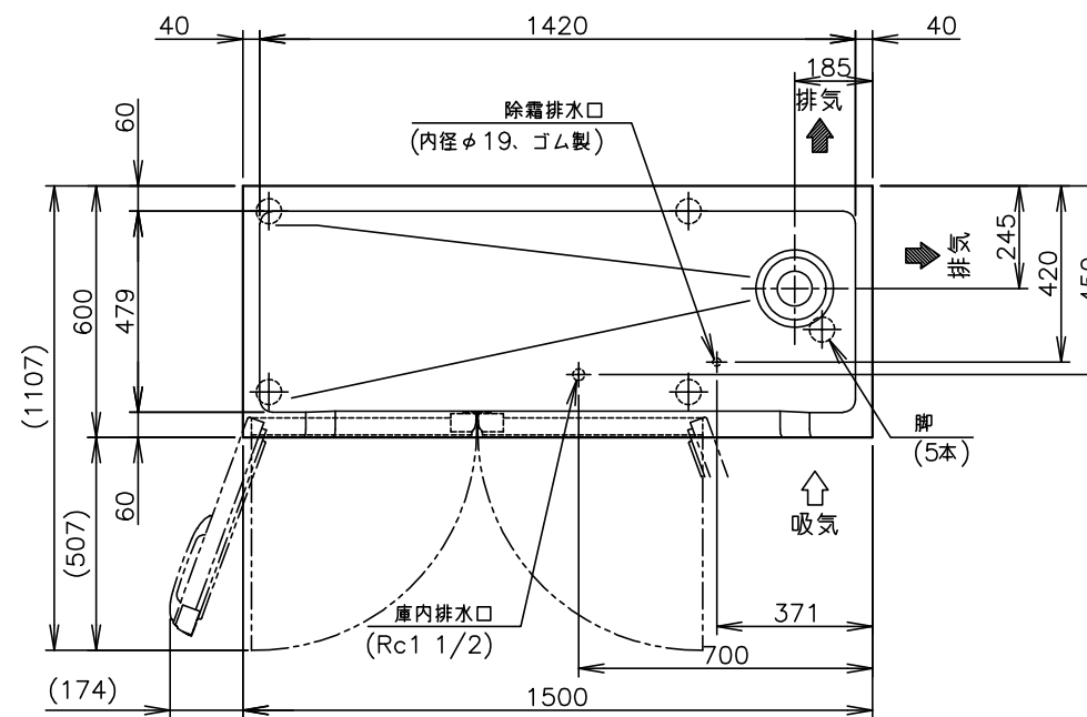
B矢視図(1/10)
