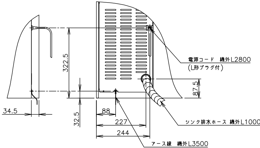
A矢視図 (1/10)
