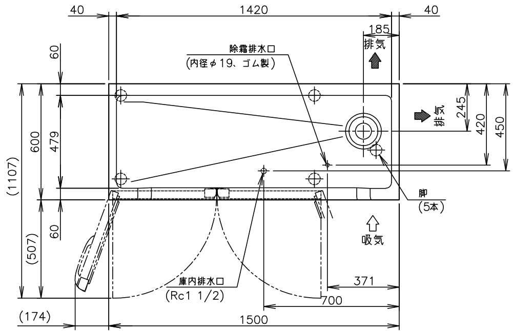
A矢視図 (1/10)
