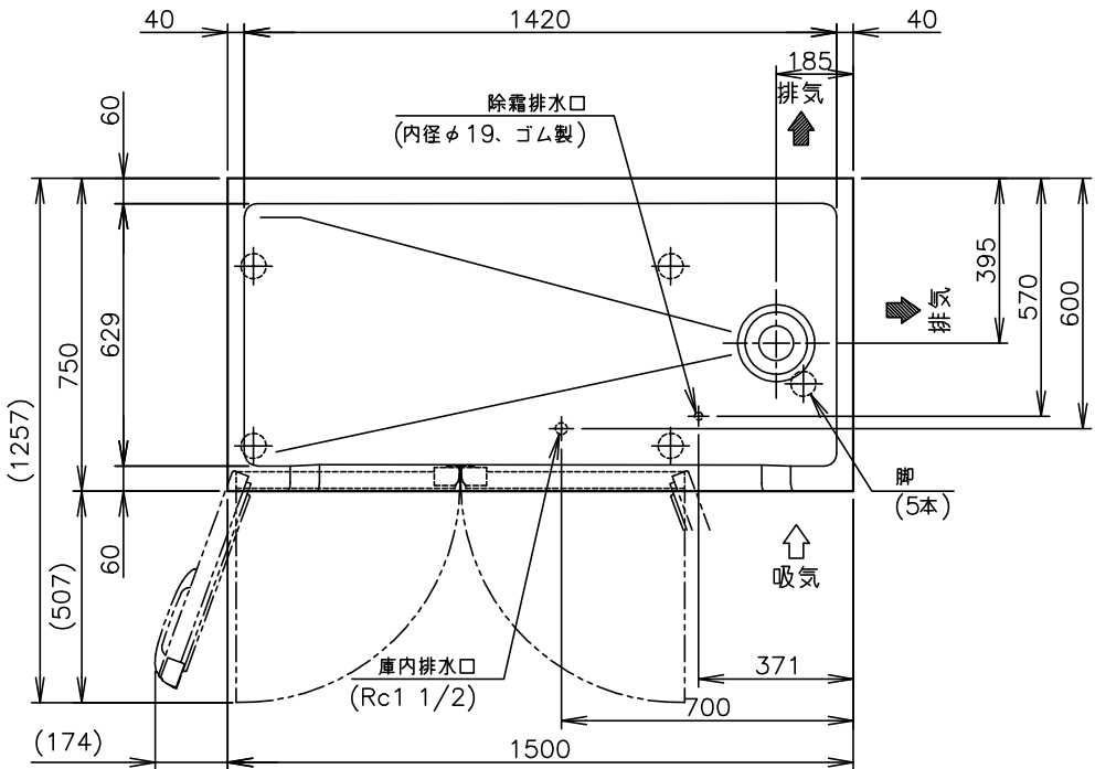
B矢視図(1/10)
