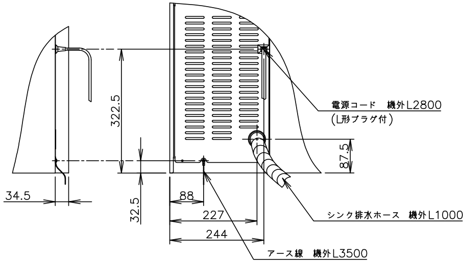
A矢視図 (1/10)
