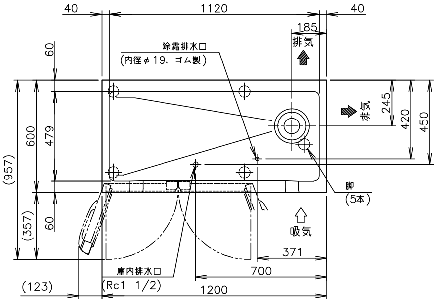
A矢視図 (1/10)
