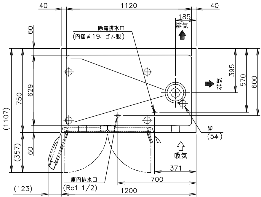
B矢視図(1/10)
