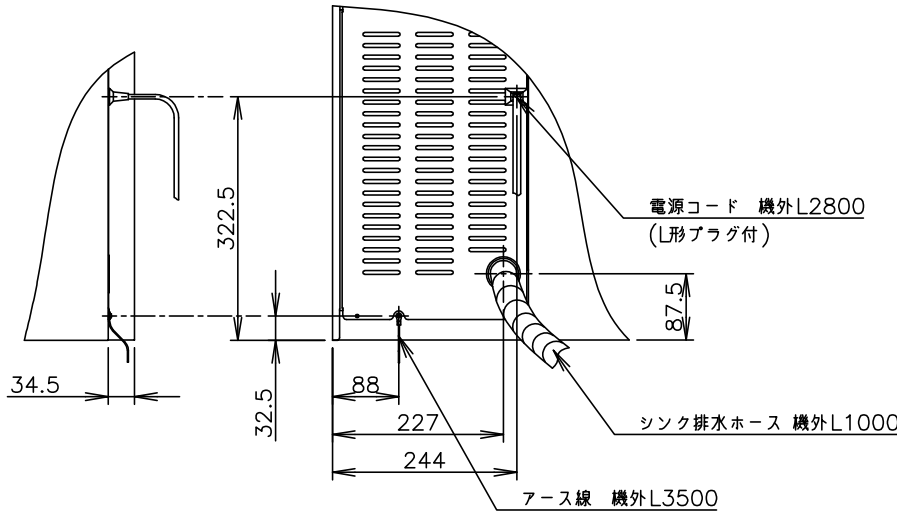
B矢視図(1/10)
