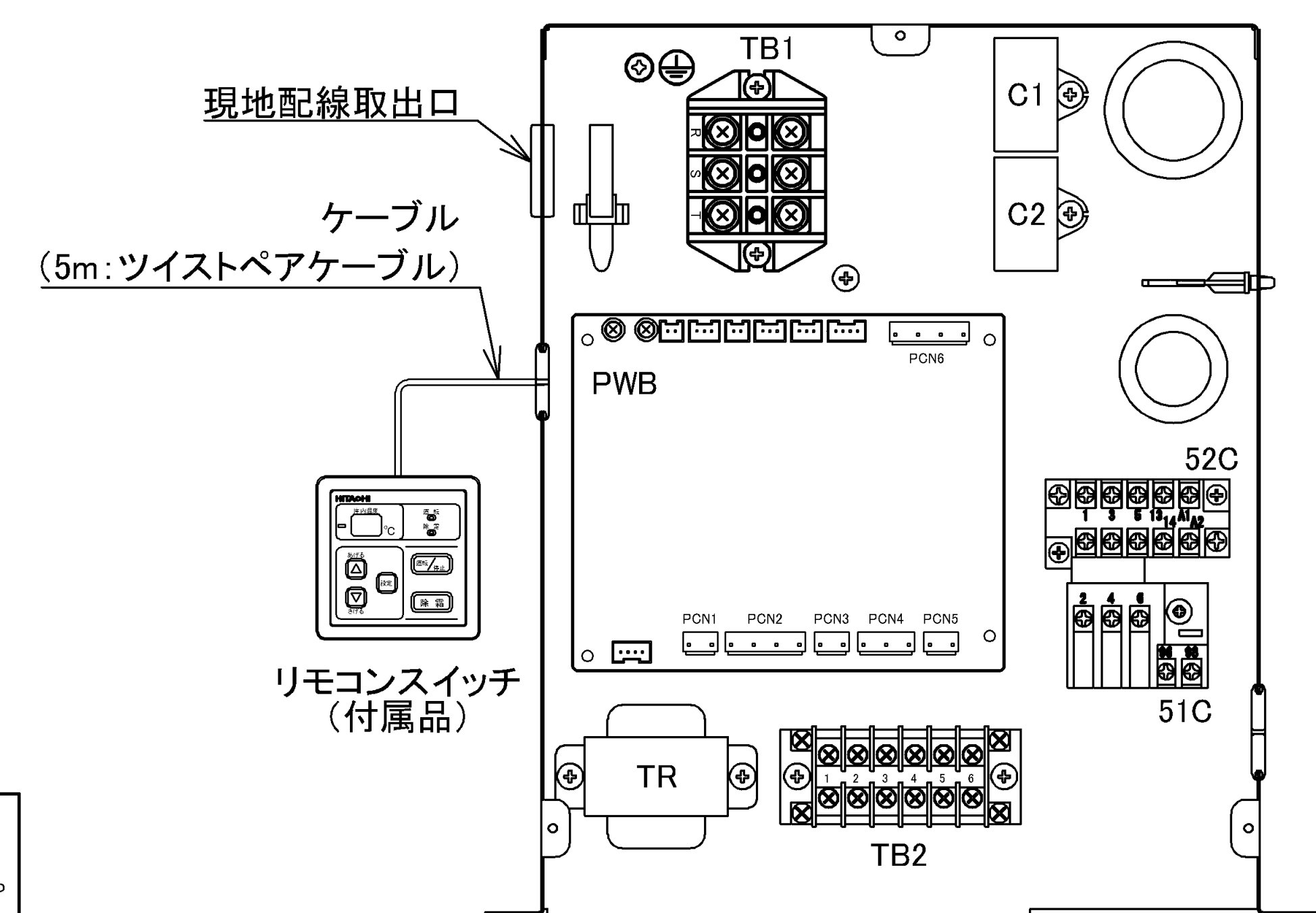
ユニット電気箱内配置図
