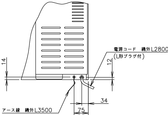
A矢视图(1/10)
