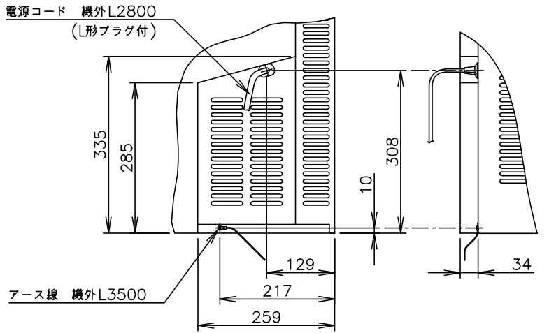
A矢视图(1/10)
