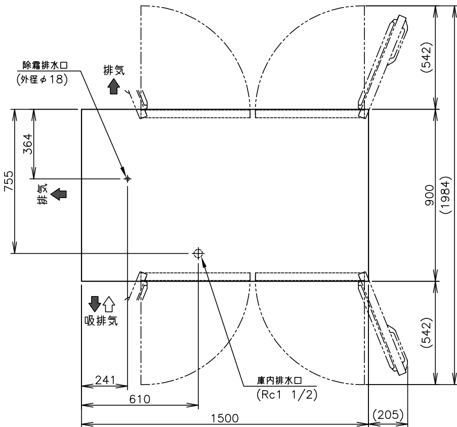
A矢视图 (1/10)
