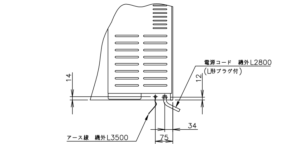
A矢视图 (1/10)
