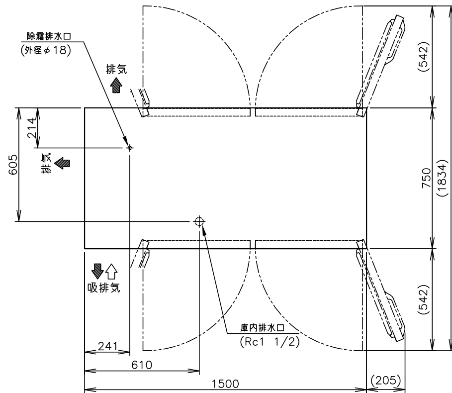
A矢視図(1/10)
