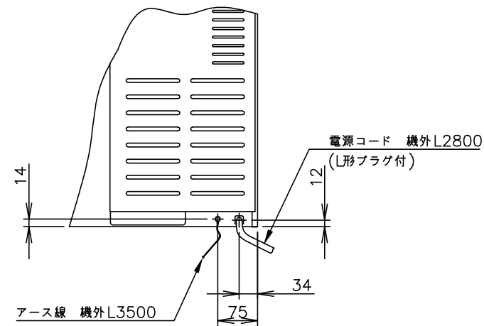
A矢視図(1/10)
