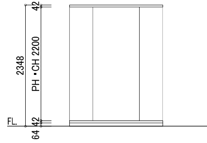
立面図B
