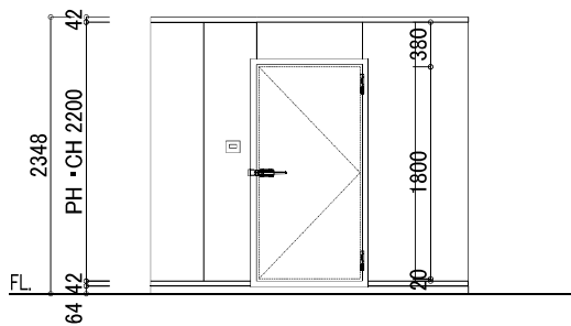
立面図A
