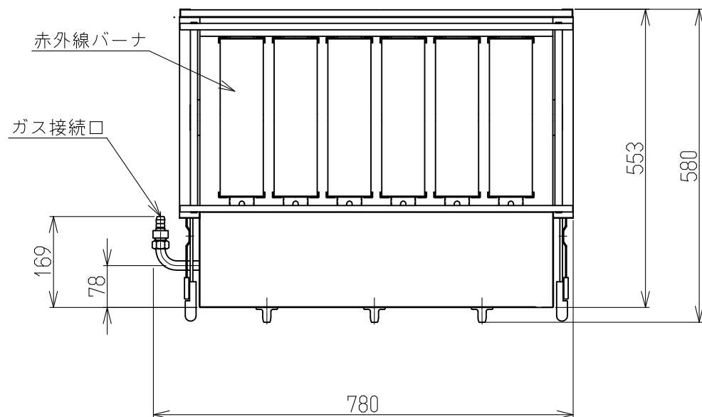
焼網寸法
