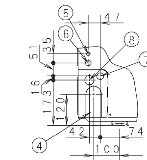
矢視図B
