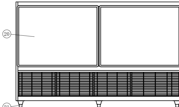
(A矢视图)
