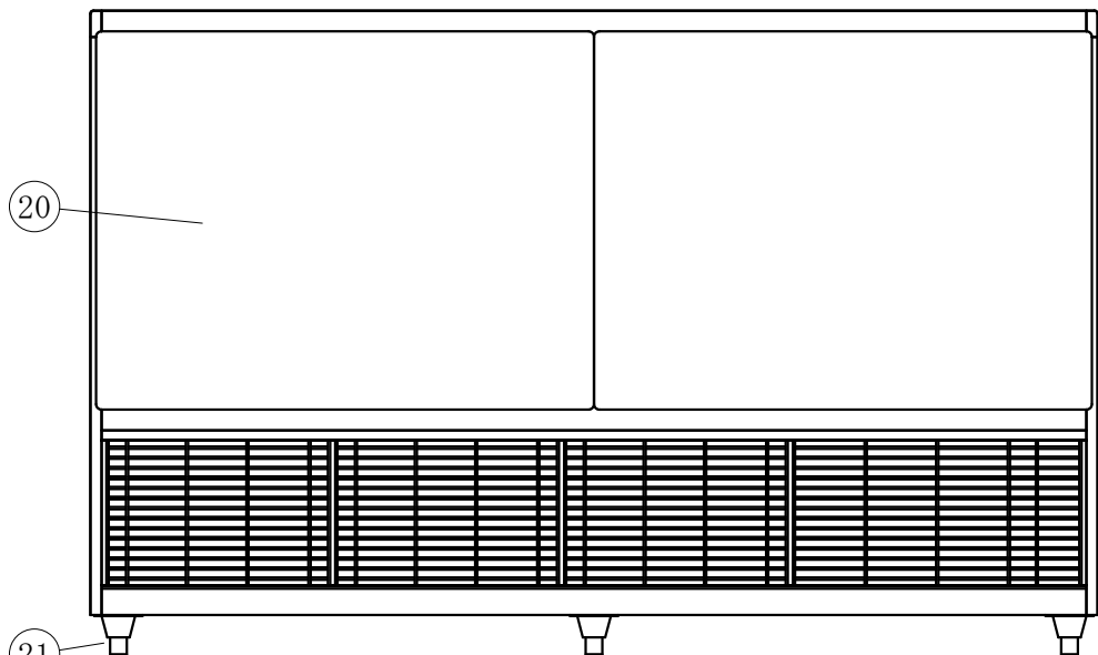
(A矢視図)
