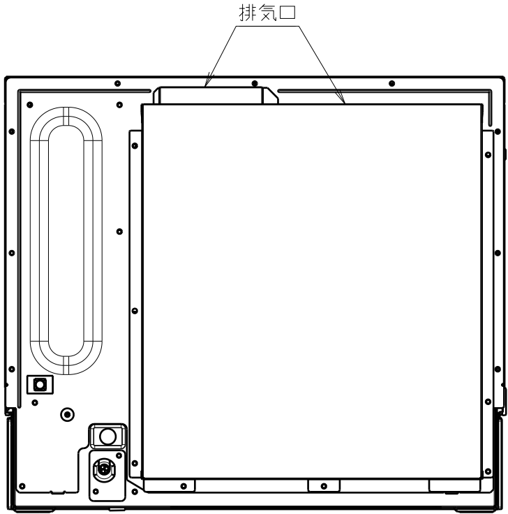
背面図
