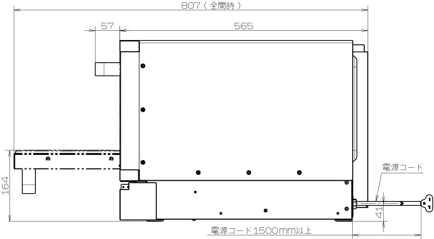
側面図
