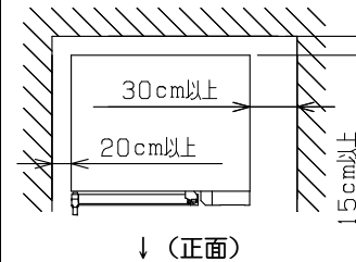
メンテナンススペース
