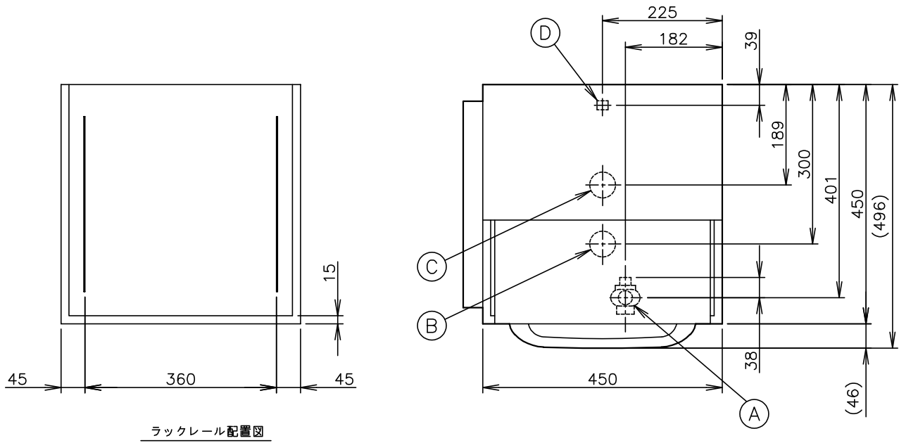
ラックレール配置図
