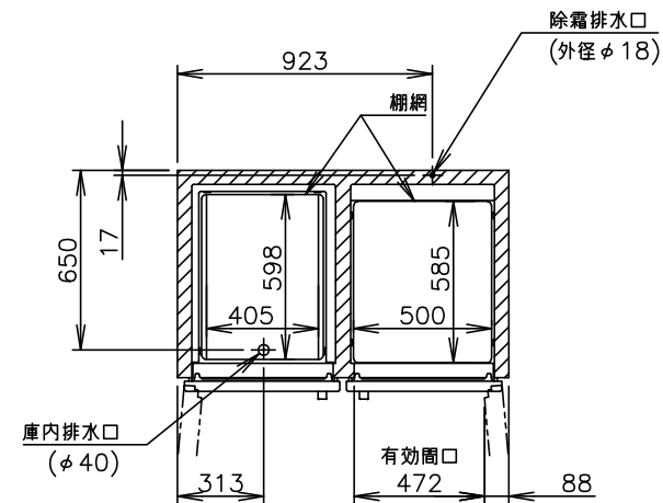
平面断面図(下室)
