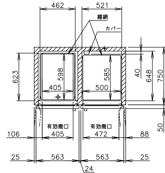
平面断面图(上室)
