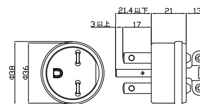
单相200Vプラグ形状 (接地極付 15A 250V)
