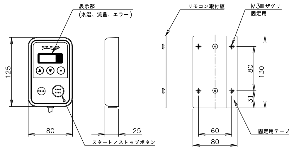
リモコン詳細図(1:4)
