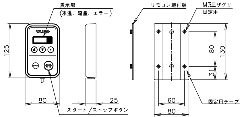
リモコン詳細図(1:4)
