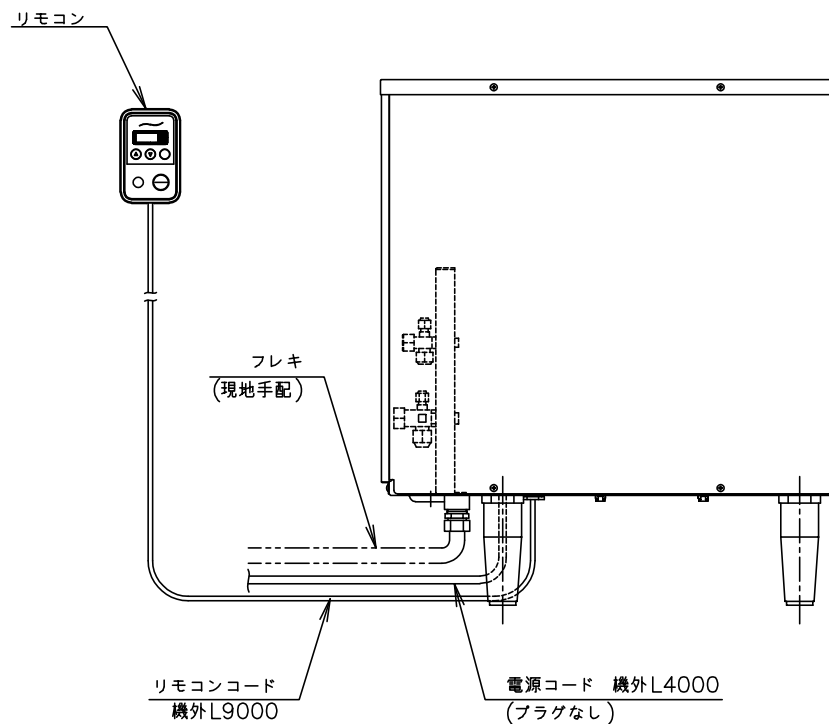
底面詳細図
