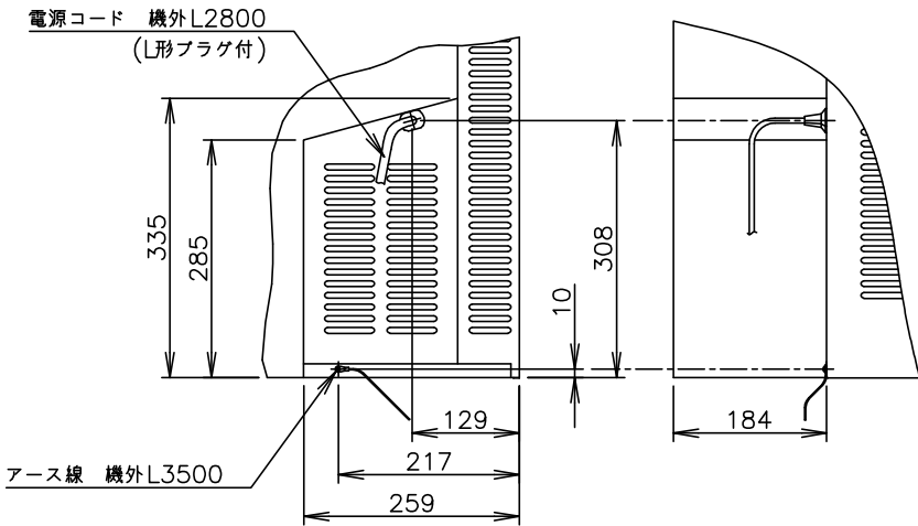
A矢视图(1/10)
