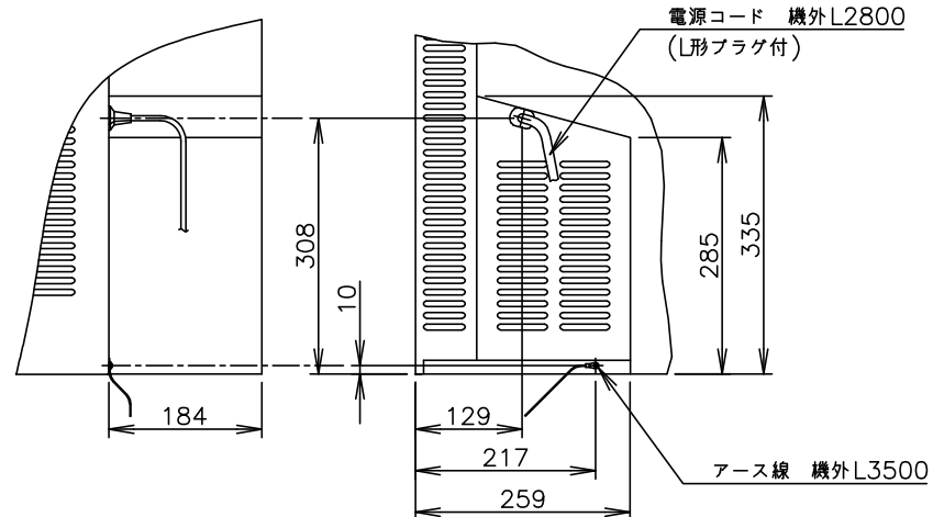
B矢視図(1/10)
