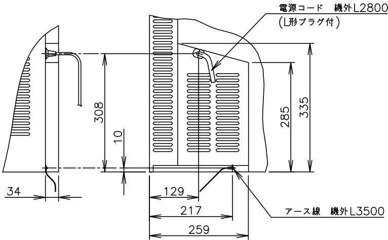
B矢視図(1/10)
