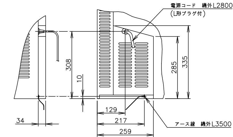
B矢视图 (1/10)
