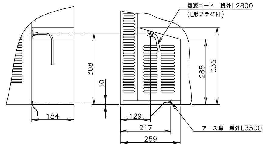
B矢視図(1/10)
