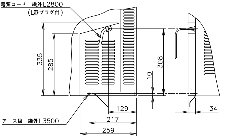
A矢视图(1/10)
