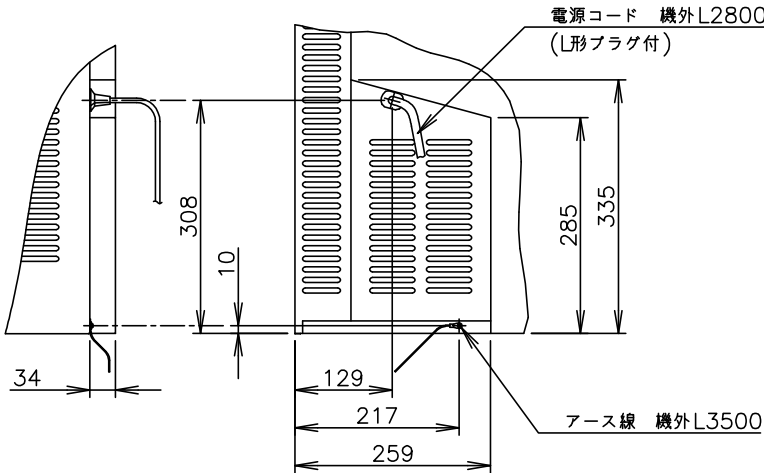
B矢视图(1/10)
