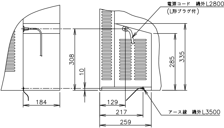
B矢視図(1/10)
