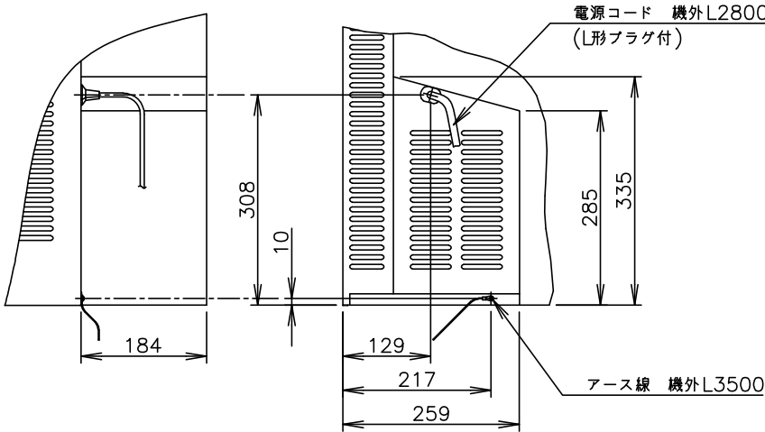
B矢視図(1/10)
