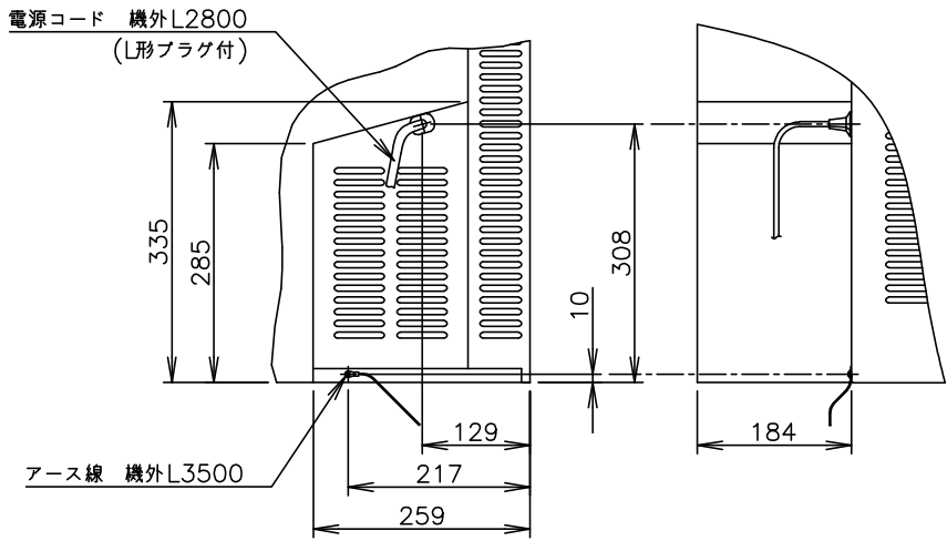
A矢视图 (1/10)
