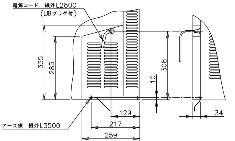
A矢视图(1/10)
