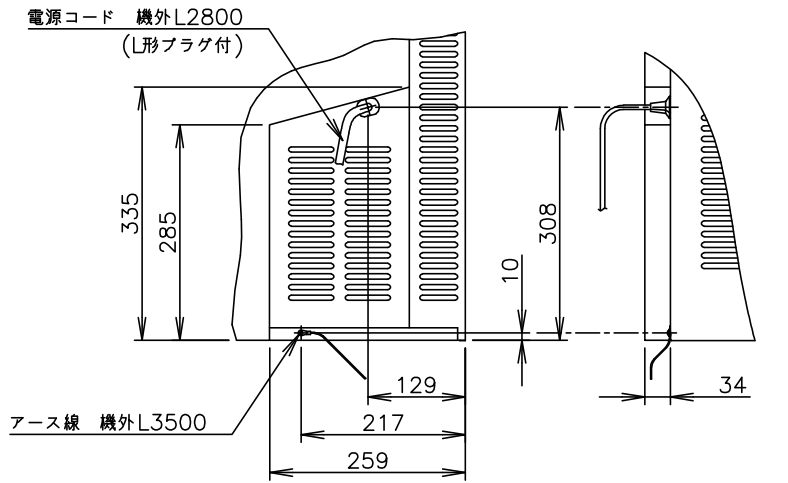
A矢视图(1/10)
