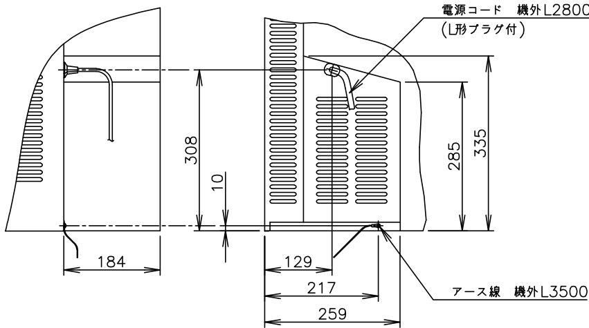
B矢视图(1/10)
