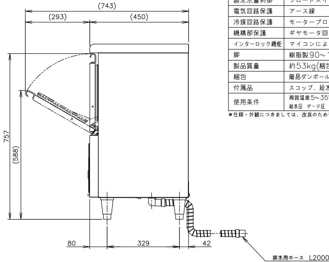
電源コード 機外L2800 (L形プラグ付)(底面)
