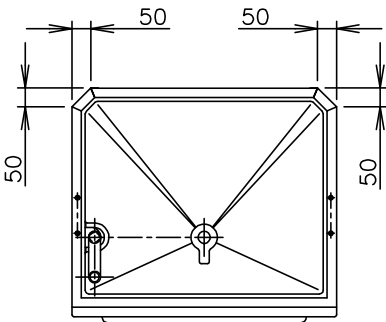
ストック上面図
