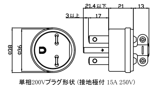
単相200Vプラグ形状 (接地極付 15A 250V)
