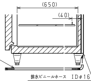
冷蔵室 排水部 (棚) 詳細
