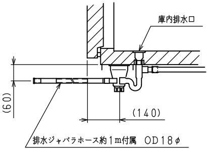
排水部詳細
